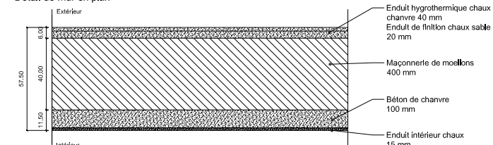
Détail de mur en plan
