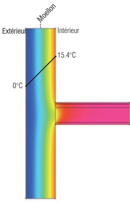
Comportement thermique du mur Existant
